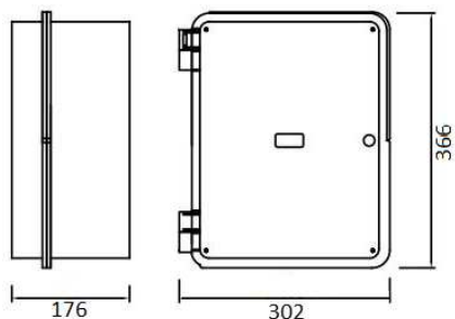
Vista Lateral
